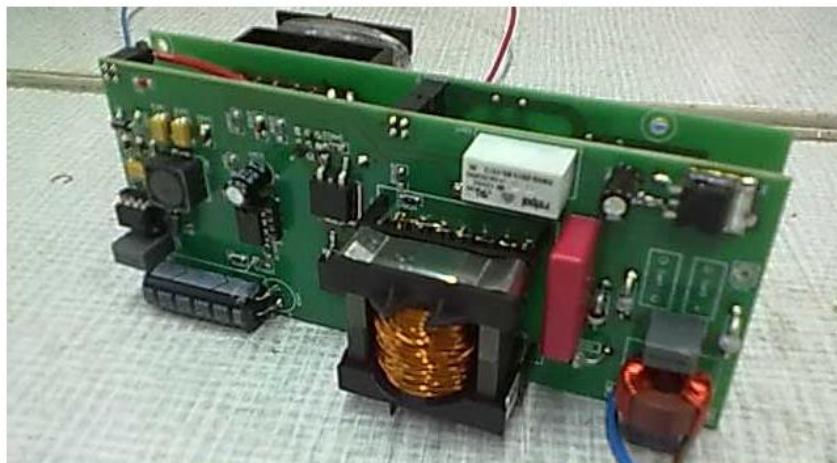
Widok opracowanego statecznika. Układ Przeciwwzakłóceńowy oraz PFC
